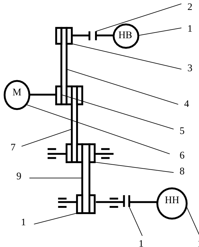
Рисунок 3.1 – Схема приводу насосів високого і низького тиску палива 1 – насос високого тиску; 2 – муфта випередження
