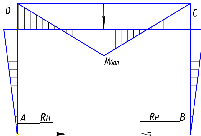
Рисунок 3.4 – Епюра згинальних моментів
