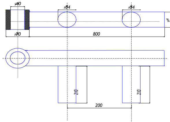
Рисунок 3.8 – Схема пристосування
